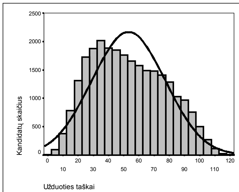
1 diagrama. Valstybinio lietuvių gimtosios kalbos brandos egzamino testo dalį laikusių kandidatų gautų taškų pasiskirstymas
