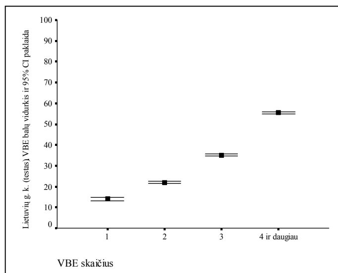
8 diagrama. Priklausomybė tarp laikytų valstybinių brandos egzaminų skaičiaus ir lietuvių gimtosios kalbos brandos egzamino testo dalies rezultatų
