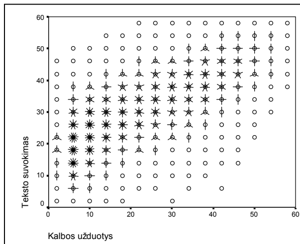
6 diagrama. Kalbos užduočių dalies ir teksto suvokimo dalies koreliacija
