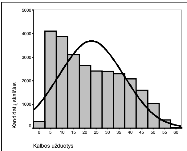
4 diagrama. Kalbos užduočių dalies taškų pasiskirstymas
