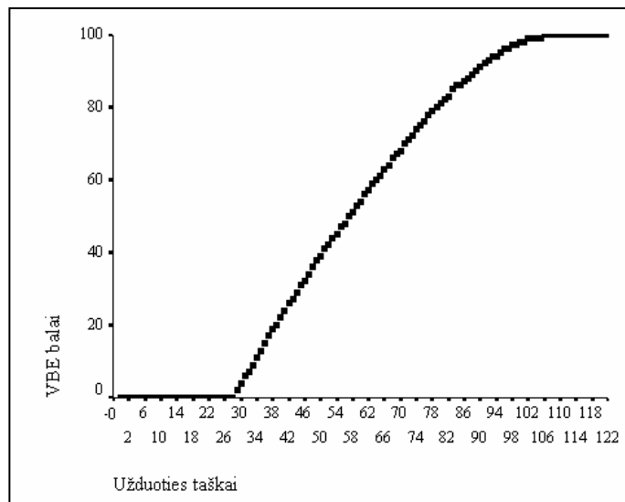
7 diagrama. Užduoties taškų ir VBE balų santykis
