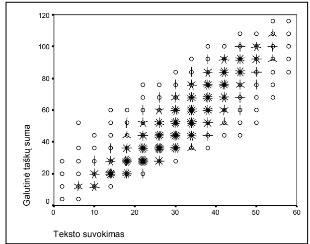
3 diagrama. Teksto suvokimo užduoties ir visos egzamino užduoties koreliacija
