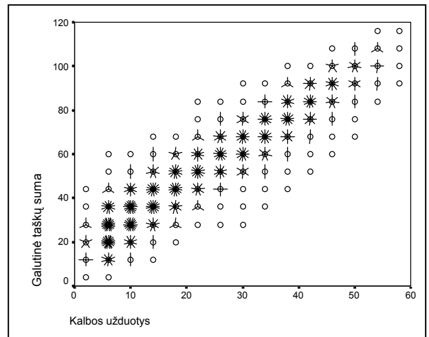
5 diagrama. Kalbos užduočių dalies ir visos egzamino užduoties koreliacija
