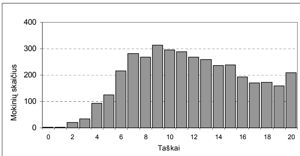
5 diagrama. Kalbos vartojimo testo taškų pasiskirstymas
