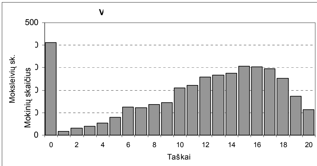
6 diagrama. Rašymo testo taškų pasiskirstymas
