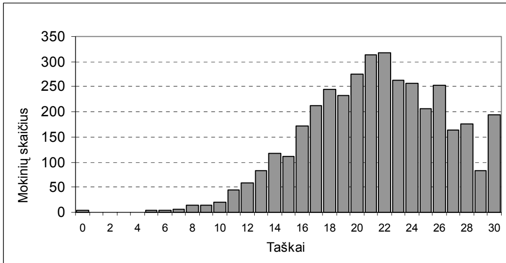
3 diagrama. Klausymo testo taškų pasiskirstymas
