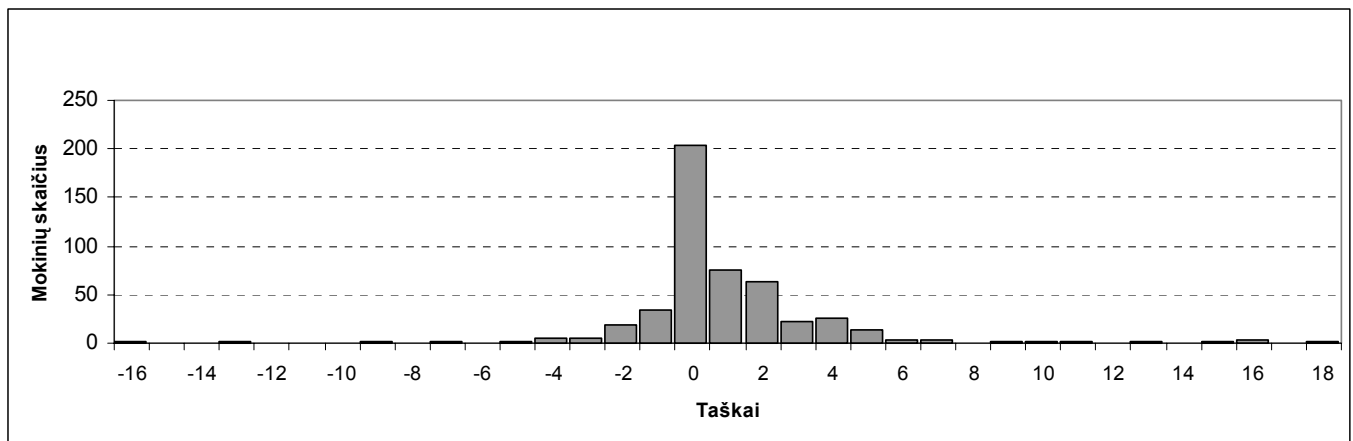
12 diagrama. Darbų imties pervertinimo statistika
