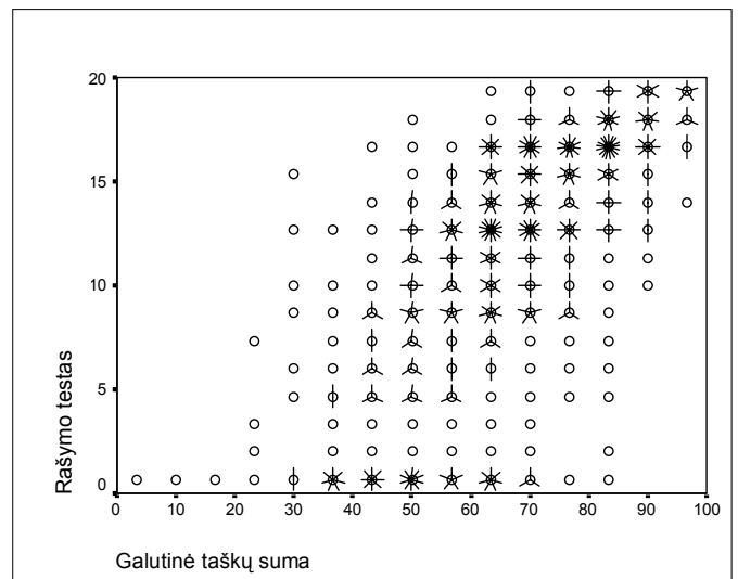
10 diagrama. Rašymo testo ir visos egzamino užduoties koreliacija (koef. 0,71)
